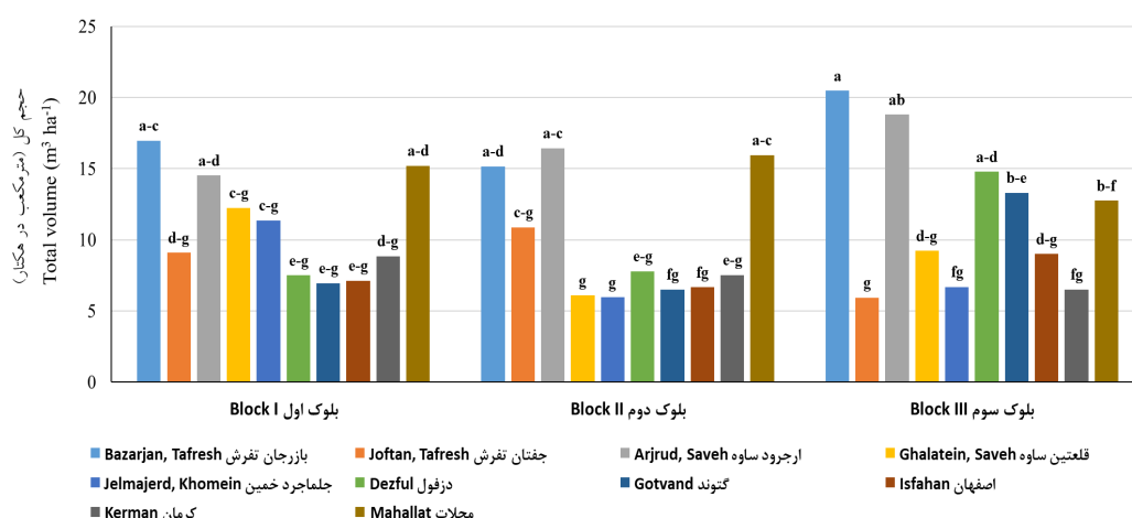
شکل ۴- میانگین متغیر حجم کل درختان پده تحت اثر متقابل رویشگاه و بلوک در سال سوم پس از کاشت با آزمون چنددامنه‌ای دانکن.
