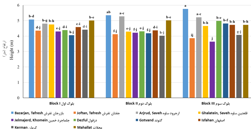
شکل ۳- میانگین متغیر ارتفاع درختان پده تحت اثر متقابل رویشگاه و بلوک در سال سوم پس از کاشت با آزمون چنددامنه‌ای دانکن. Figure 3. Mean height of Populus euphratica trees under the interaction effect of site × block in the third year after planting using Duncan's multiple range test.
