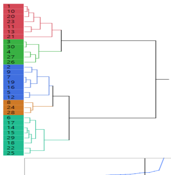
شکل ۵- دندروگرام تحلیل خوشه‌بندی سلسله‌مراتبی صفات رشدی درختان پده با استفاده از روش Ward.
