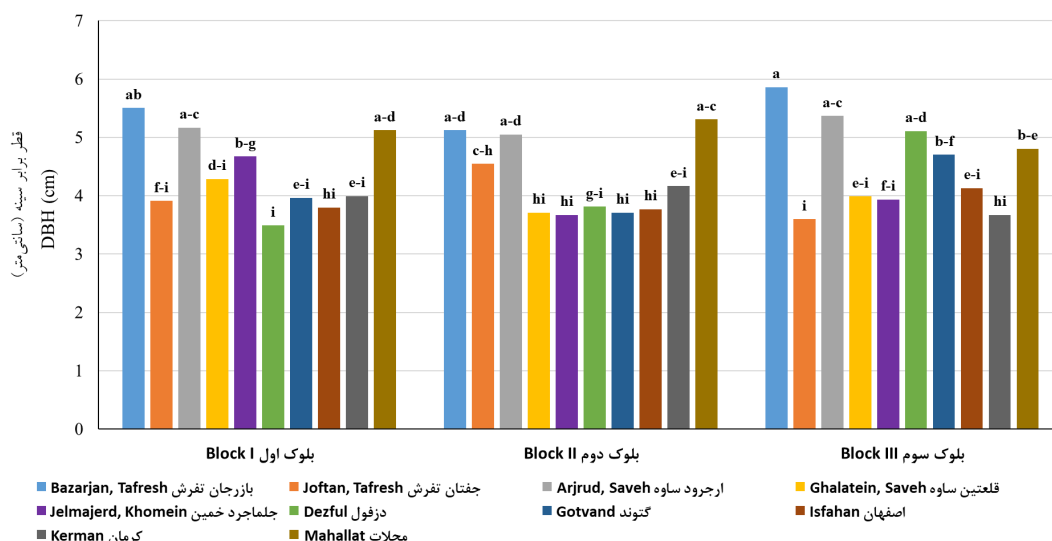
شکل ۲- میانگین متغیر قطر برابر سینه درختان پده تحت اثر متقابل رویشگاه و بلوک در سال سوم پس از کاشت با آزمون چنددامنه‌ای دانکن.
