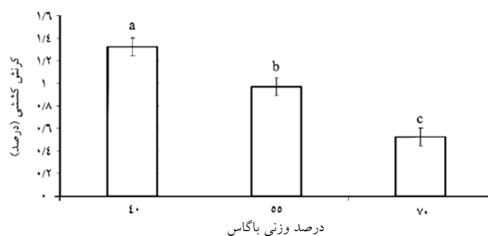
شکل ۱۲- اثر مستقل مقدار الیاف بر کرنش کششی چندسازه‌های حاوی باگاس - پلی‌پروپیلن.
