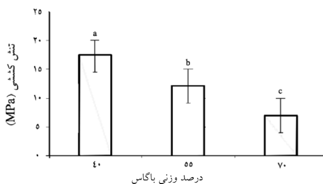
شکل ۲- اثر مستقل مقدار الیاف بر تنش کششی چندسازه های باگاس - پلی پروپیلن.
