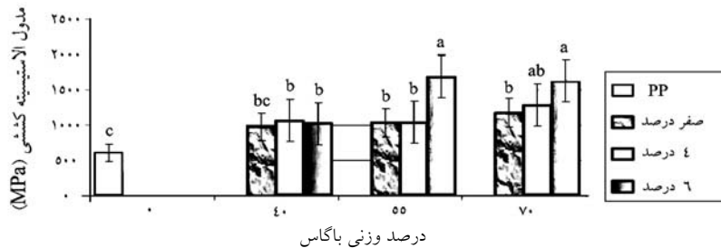
شکل ۴- مقایسه تغییرات مدول کششی چندسازه‌ها با پلی‌پروپیلین خالص.
