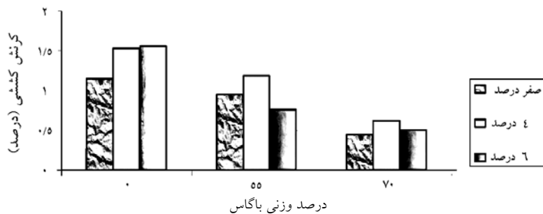
شکل ۱۴- اثر متقابل مقدار باگاس و مقدار سازگارکننده بر کرنش کششی چندسازه‌های باگاس - پلی‌پروپیلن.
