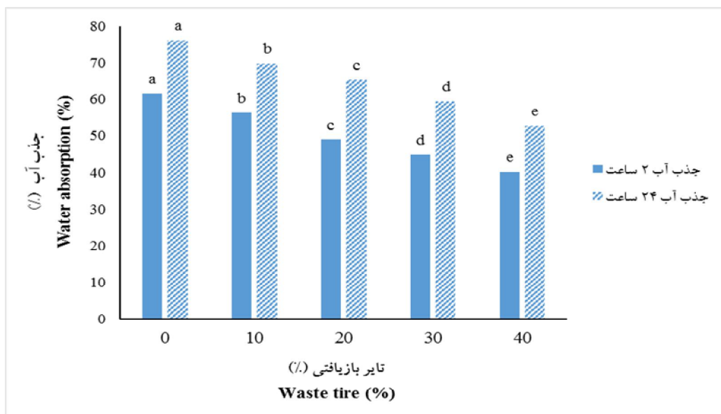
شکل ۴- تأثیر سطوح مختلف تایلر بازیافتی بر جذب آب بعد از ۲ و ۲۴ ساعت غوطه‌وری در آب.
