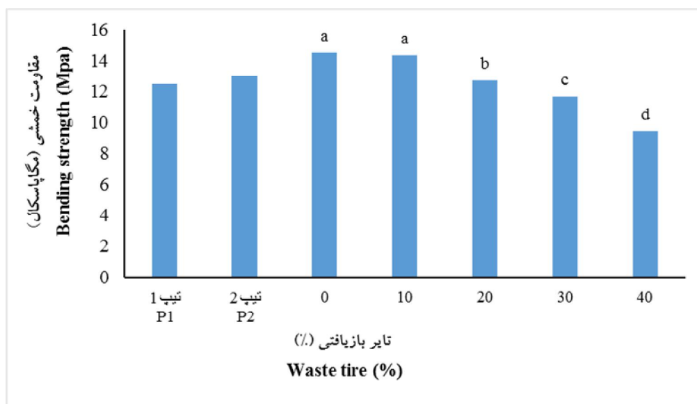
شکل ۱- تأثیر سطوح مختلف تایر بازیافتی بر مقاومت خمشی.
