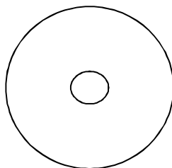
شکل ۲- قطعات دایره‌ای شکل متحدالمركز، مساحت دایره بزرگ ۱۰۰۰ مترمربع و دایره کوچک ۴ مترمربع می‌باشد. Figure 2. Concentric circular plots, the area of the large and small circles is 1000 m 2 and 4 m 2 , respectively.
