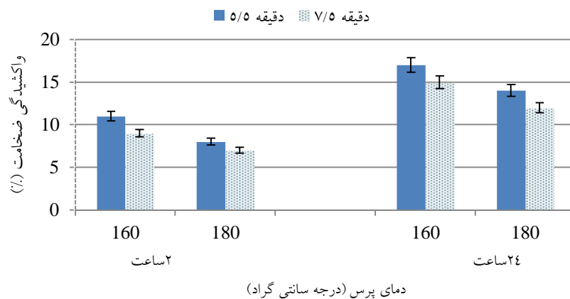
شکل ۴- خواص فیزیکی تخته خرده‌چوب ساخته شده با رزین تانن اپوکسی اکریلات. Figure 4. Physical Properties of Particleboard with Tannin Epoxy Acrylate Resin.
