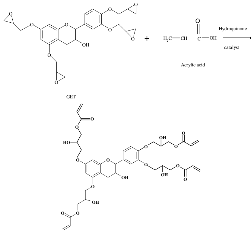
طرح ۱- فرایند سنتز رزین تانن اپوکسی اکریلات.
