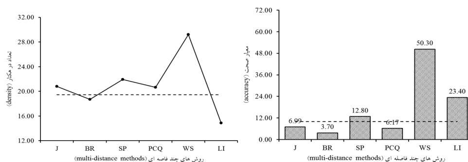
شکل ۵- مقایسه تعداد در هکتار برآورد شده توسط روش‌های چندفاصله‌ای ترکیبی (J)، بایت و رایپلی (BR)، نقطه مشترک (SP)، مربعی با نقطه مرکزی (PCQ)، مربع سرگردان (WS) و برخورد خطی (LI) و معیار صحت آن‌ها (خط چین نشان‌دهنده مقدار واقعی تراکم (۱۹/۴۴ پایه در هکتار) و درصد قابل قبول معیار صحت (۱۰ درصد) می‌باشد).
