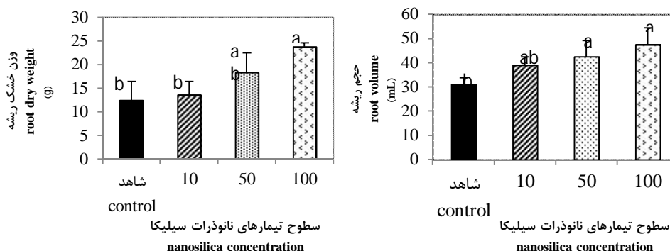
شکل ۳- مقایسه میانگین حجم و وزن خشک ریشه گونه زالزالک ( C. aronia ) تحت تأثیر نانوذرات سیلیکا با استفاده از آزمون Dunnett's T3 در سطح اطمینان ۹۵ درصد.
