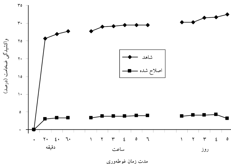
شکل ۴- مقایسه مقدار واکشدگی ضخامت تخته خرده باگاس اصلاح شده و نمونه شاهد.
