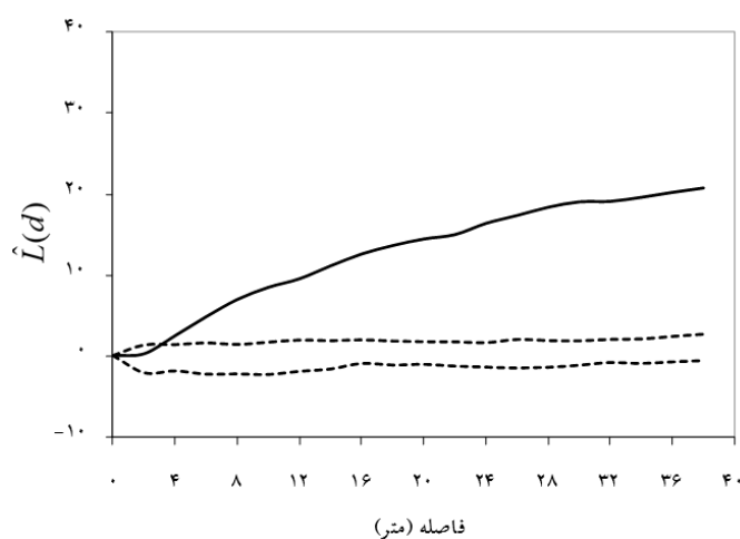
شکل ۹- الگوی مکانی درختان بنه با استفاده از تابع استاندارد شده رایبلی. خط ممتد نشان‌دهنده مقادیر \hat{L}(d) و خطوط بریده حدود اعتماد مونت کارلو هستند.
