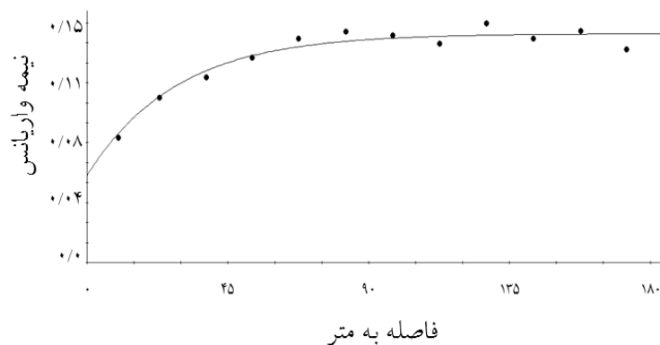
شکل ۵- واریوگرام تجربی و مدل نمایی برازش شده.
