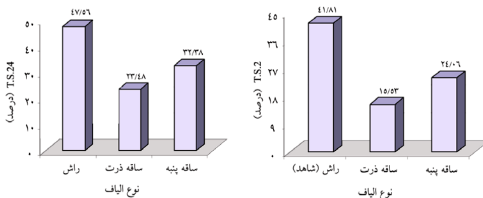
شکل ۶- اثر نوع الیاف بر واکنش‌پذیری ضخامت ۲ و ۲۴ ساعت تخته فیبر دانسیته متوسط.
