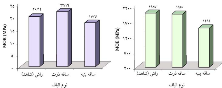
شکل ۲- میانگین مقاومت خمشی و مدول الاستیسیته تخته‌های ساخته شده در دمای ۱۸۰ درجه سانتی‌گراد.
