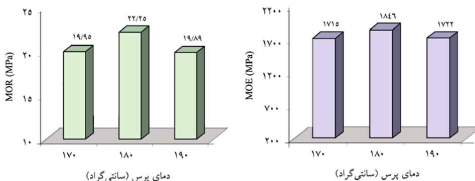
شکل ۳- میانگین مقاومت خمشی و مدول الاستیسیته تخته‌های ساخته شده از ساقه پنبه و ذرت در دماهای مختلف.
