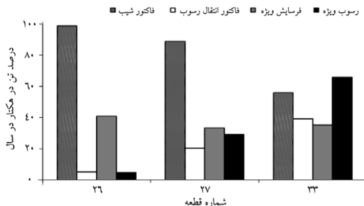
شکل ۳- تغییرات فرسایش ویژه، رسوب انتقالی ویژه، فاکتور شیب و فاکتور انتقال رسوب در قطعات مختلف.
