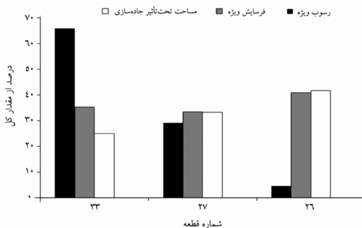
شکل ۲- تغییرات درصد از مقدار کل مساحت تحت‌تأثیر قرار گرفته، رسوب ویژه و فرسایش ویژه در قطعات مختلف.
