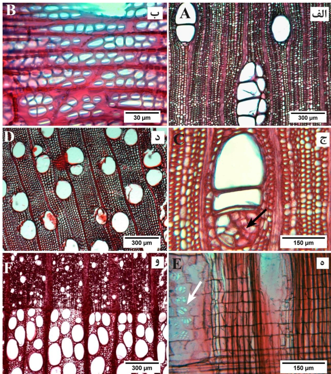
شکل ۴- مقطع عرضی چوب ناشناس موسوم به «راش روسی» (الف)، منافذ با هاله تحلیل رفته (ب) و بلور داخل تیل (فلش) (ج) در این گونه؛ مقطع عرضی (د) و شعاعی (ه) چوبی که به اشتباه «کروئینگ» نامیده شده بود، عدم وجود کانال‌های بین سلولی در مقطع عرضی (د) و نوع منافذ بین آوند و اشعه (فلش) با ویژگی‌های گونه «کروئینگ» مطابقت ندارد؛ مقطع عرضی گونه سنجد (و).
