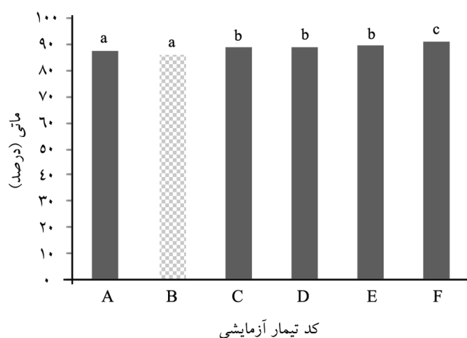
شکل ۲- تغییرات ماتی کاغذهای دست‌ساز به دست آمده از تیمارهای آزمایشی.
