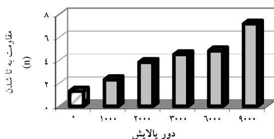
شکل ۶- مقاومت به تا شدن کاغذهای بازیافتی حاصل از روزنامه باطله در دور پالایش‌های متفاوت.
